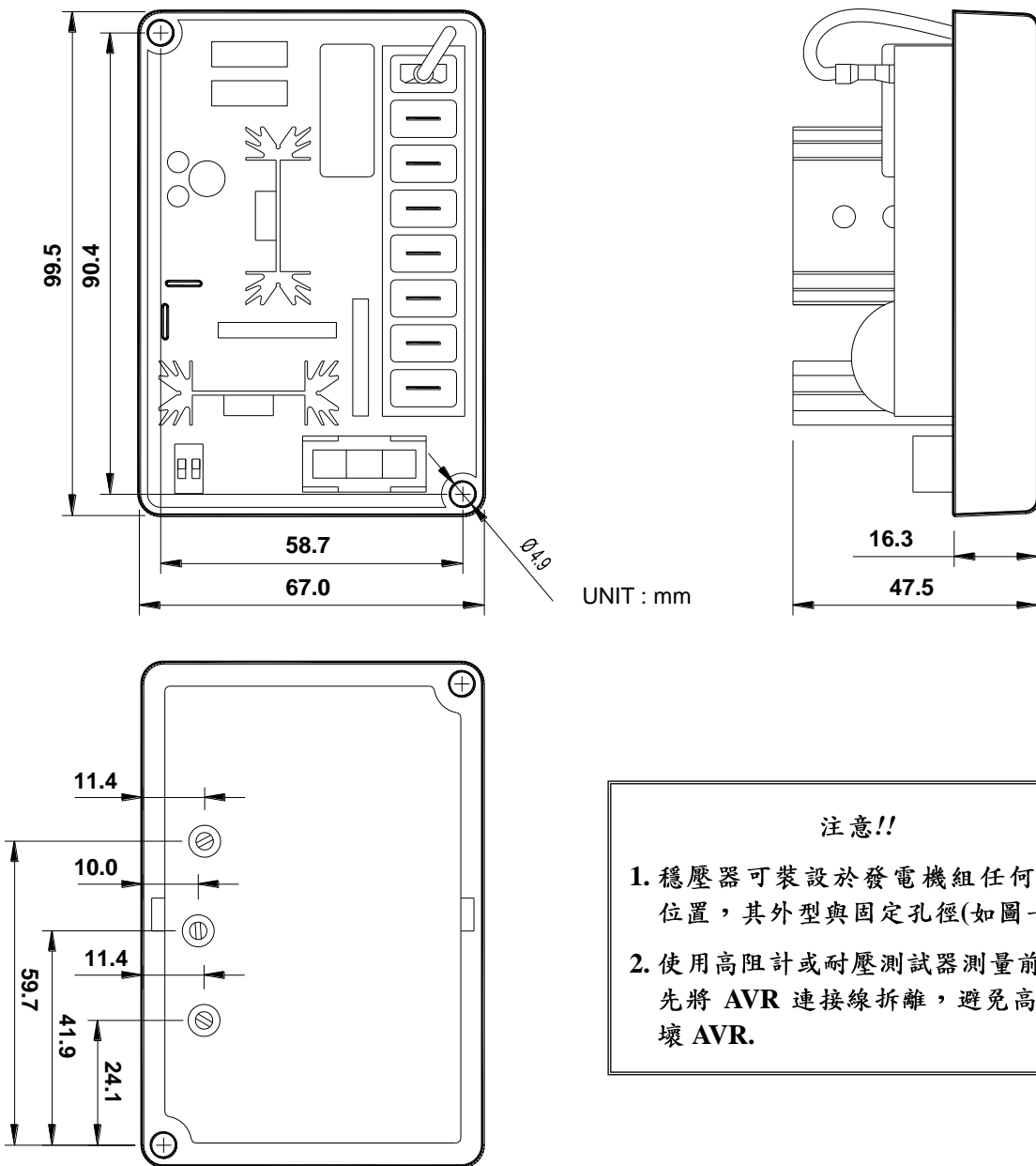
圖一 尺寸圖
